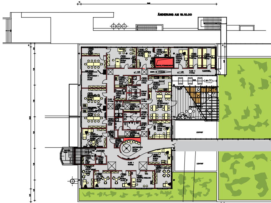
PSYCHIATRISCHE TAGESKLINIK GRUNDRISS
